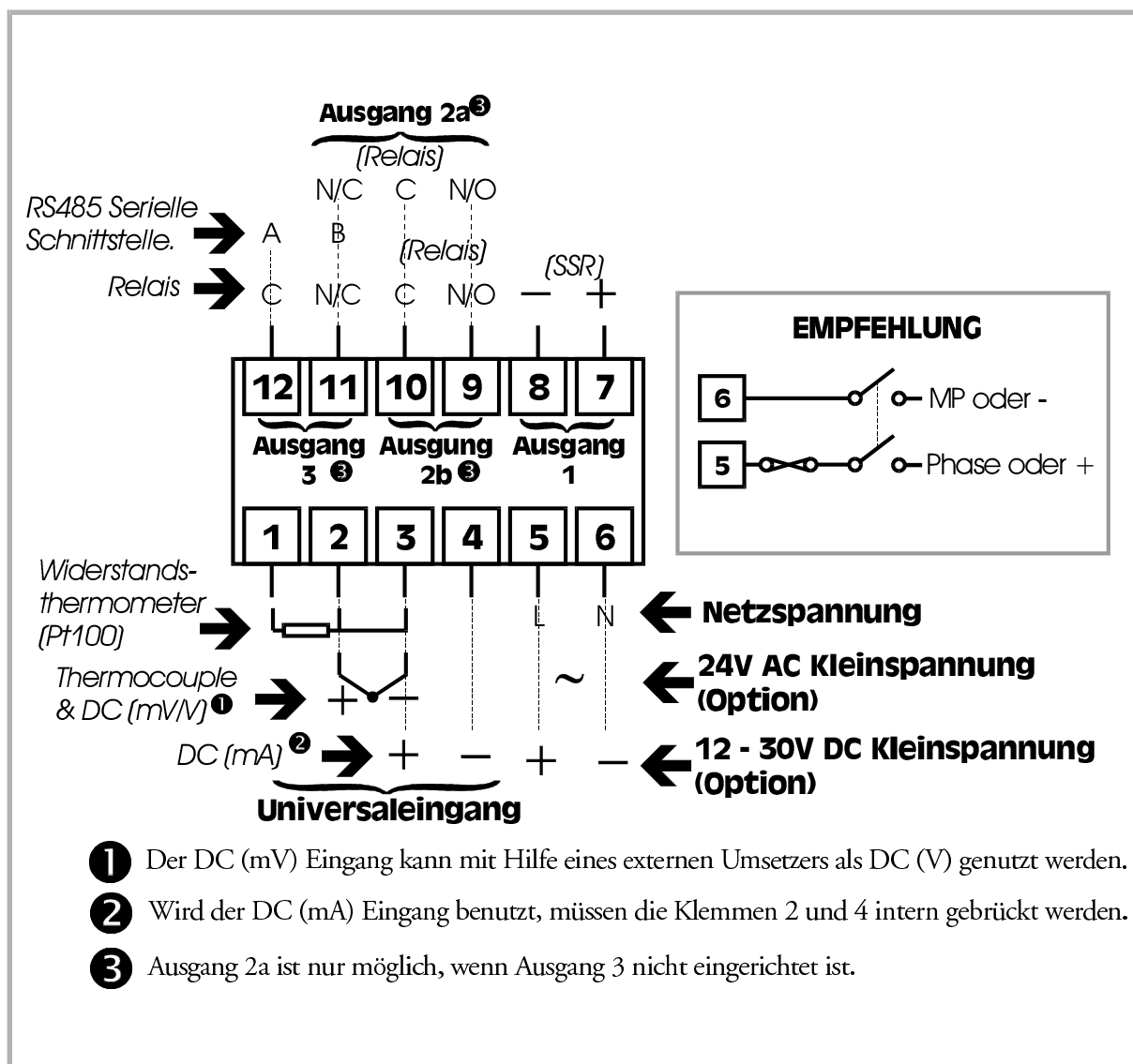
Abb. 3-1 Anschlußklemmenbelegung
